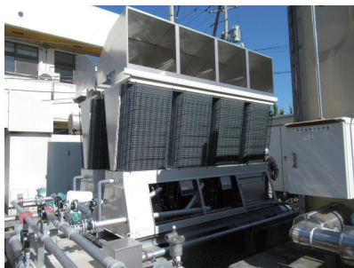
空冷ヒートポンプチラー
