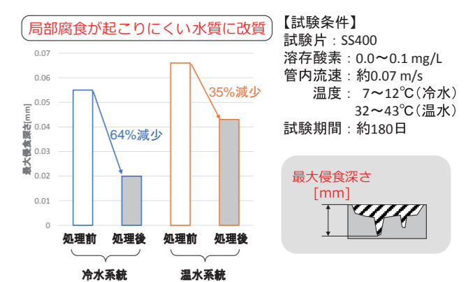
図7 アニオン交換処理前後の最大侵食深さ
