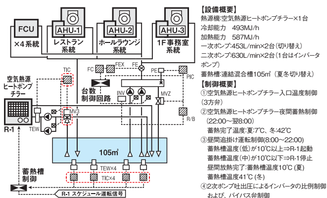
【図1】蓄熱式空調システム概要
