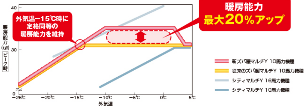
■暖房能力比較
