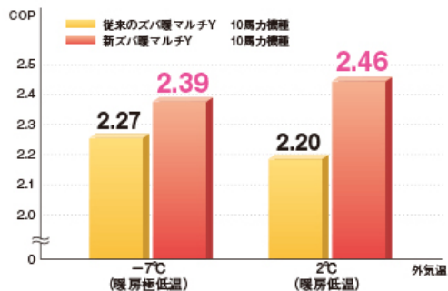
■低外気温時の省エネ性
