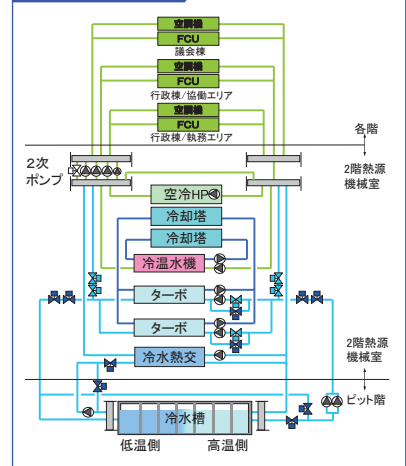
熱源システム系統図
